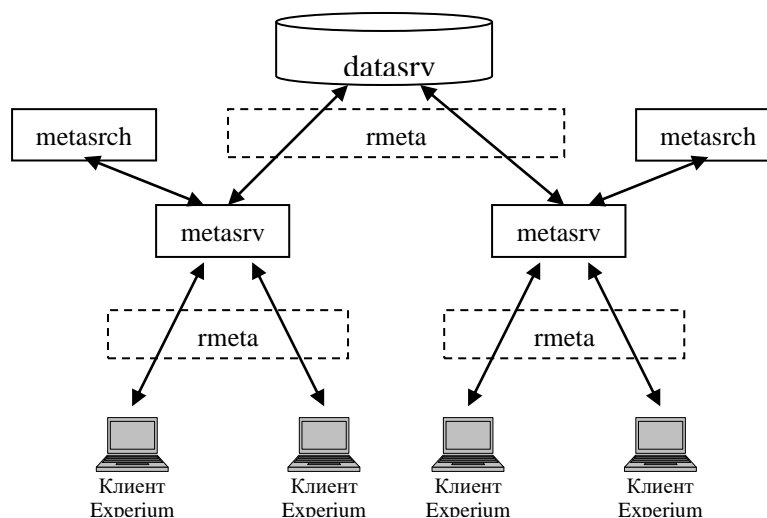
исунок 4.1. Схема компонентов программного комплекса
